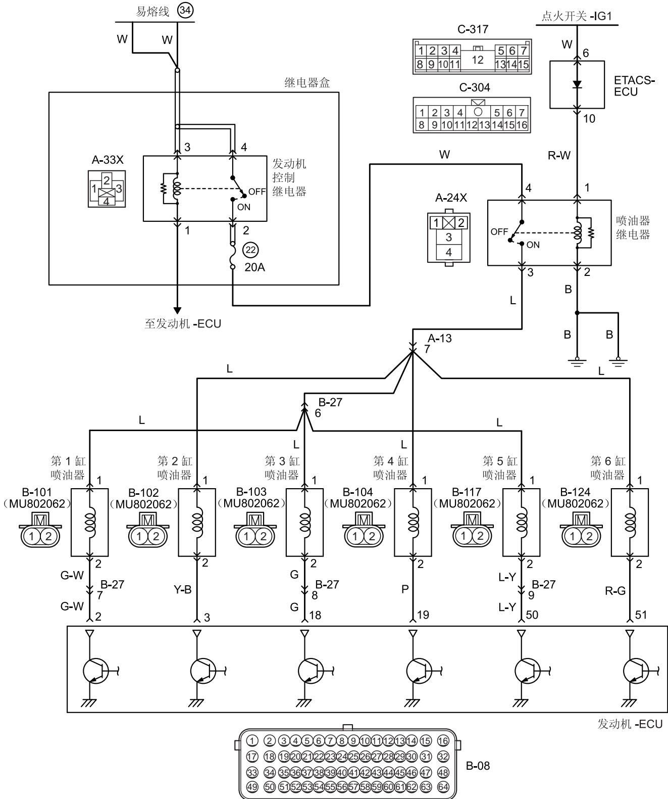
喷油器电路
